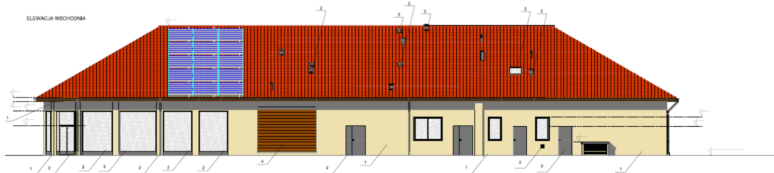
ELEWACJA PÓŁNOCNA
